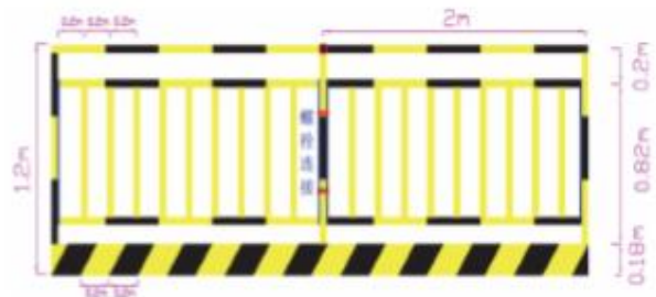
装配式固定防护栏杆示意图
